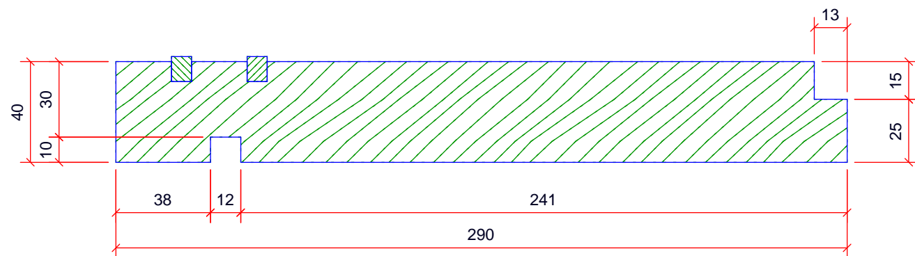
DOORSNEDE TREDE - SCHAAL 1:2
